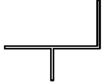
2048 ALÜMİNYUM PROFİL 0,265 Kg/m
