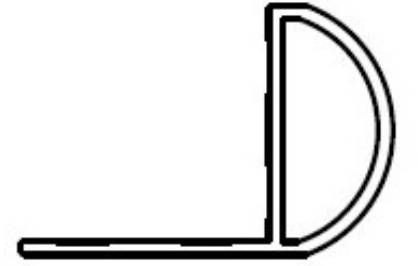
2056 20 MM MERMER PROFİLİ 0,204 Kg/m
