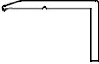
5097 ALÜMİNYUM PROFİL 0,083 Kg/m
