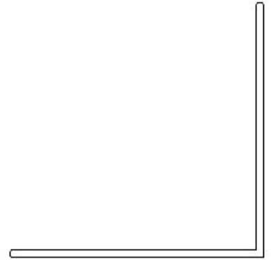
5110 ALÜMİNYUM PROFİL 0,256 Kg/m
