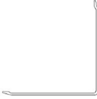
2046-1 40x40 L KÖŞE KORUMA 0,18 Kg/m
