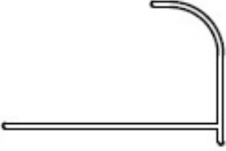
1017 12 MM LÜKS DIŞ KÖŞE PROFİLİ 0,071 Kg/m
