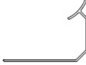
1007 10 MM İÇ KÖŞE PROFİLİ 0,045 Kg/m
