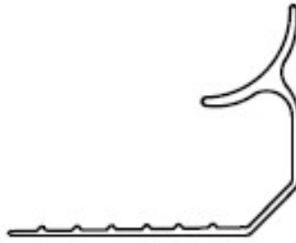
1020 10 MM YARIMAY PROFİLİ İÇ KÖŞE 0,1 Kg/m
