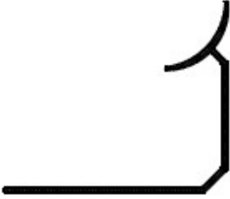
1009 14 MM İÇ KÖŞE PROFİLİ 0,087 Kg/m
